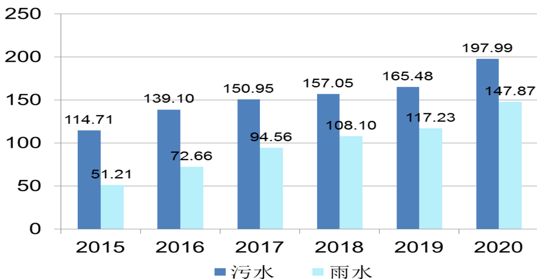
图7 “十三五”期间雨污水管道(km)增长情况图
