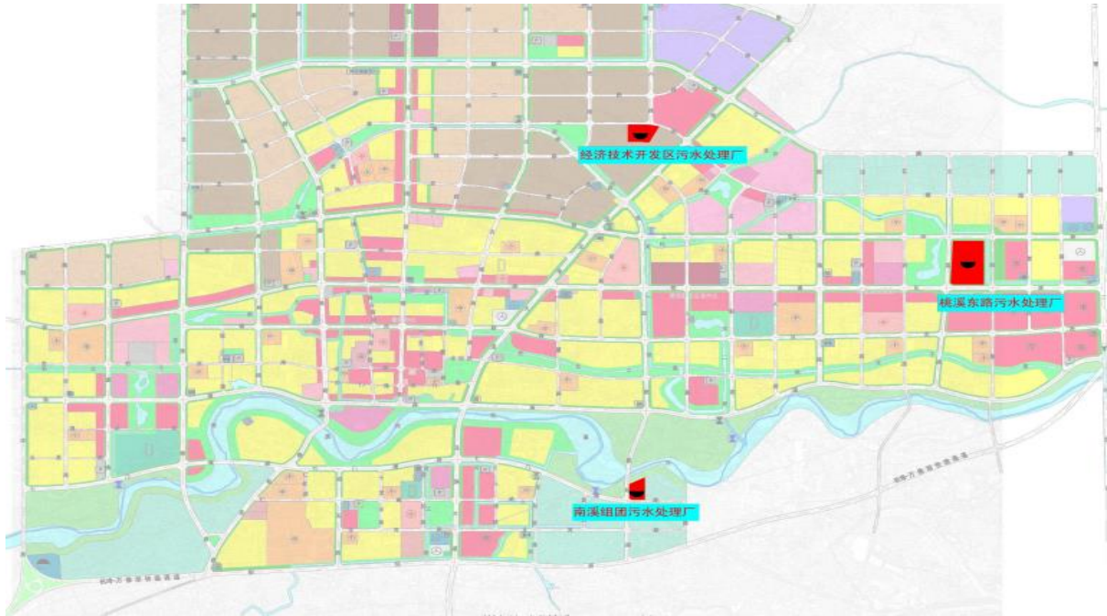
图 25 城区污水处理厂布局规划图
