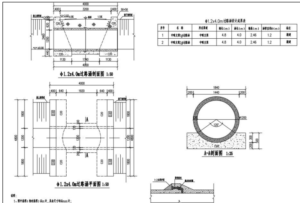
图 2-5 过路涵平面图
