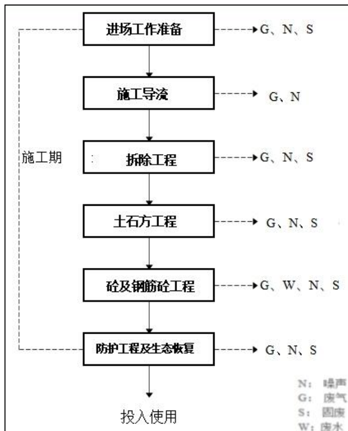
图 2-7 拦水坝施工工艺流程及产污节点图
