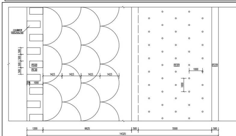
图 2-1 杨家畝拦水坝设计图
