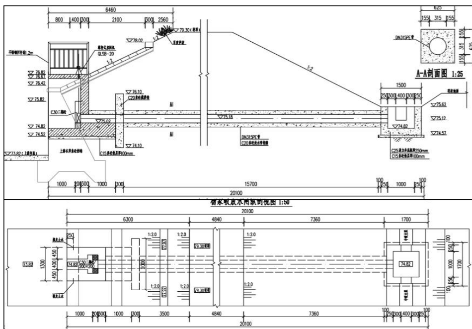
图 2-4 放水闸设计图
