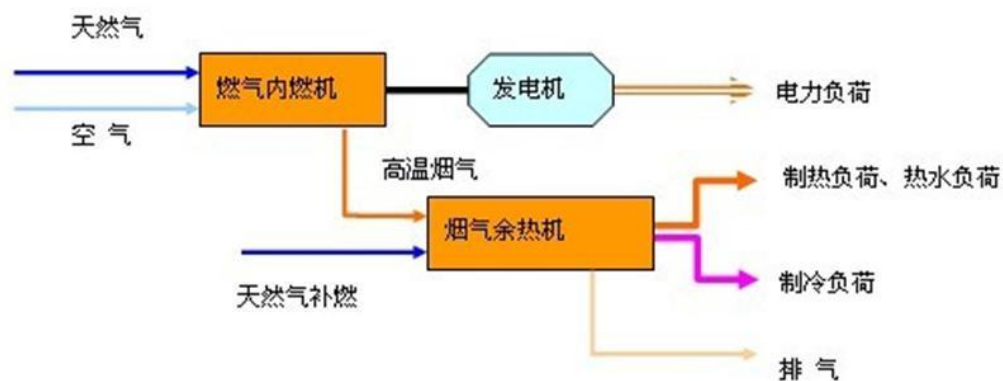
典型冷热电联产系统示意图
