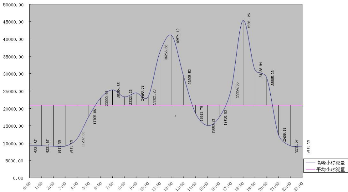
2035年舒城县城24小时用气曲线
