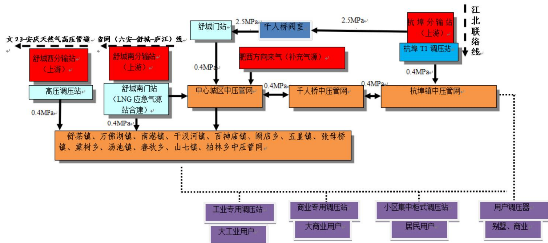
舒城县管输燃气输配系统规划图
