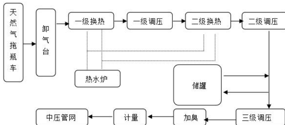
CNG 城镇供应站工艺流程图
