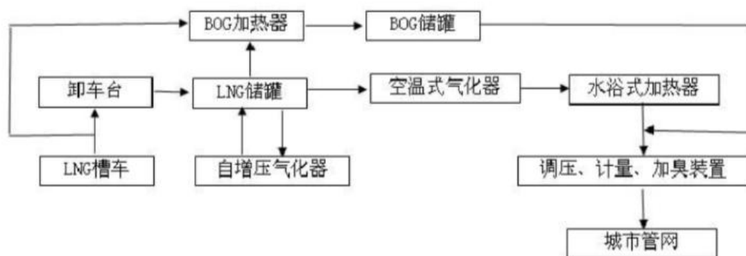
LNG 气化站工艺流程图
