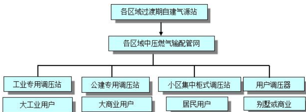
舒城县域过渡期及自建气源站区域燃气输配系统工艺流程
