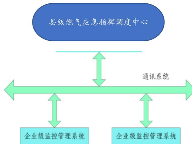
县级燃气监控管理系统框架
