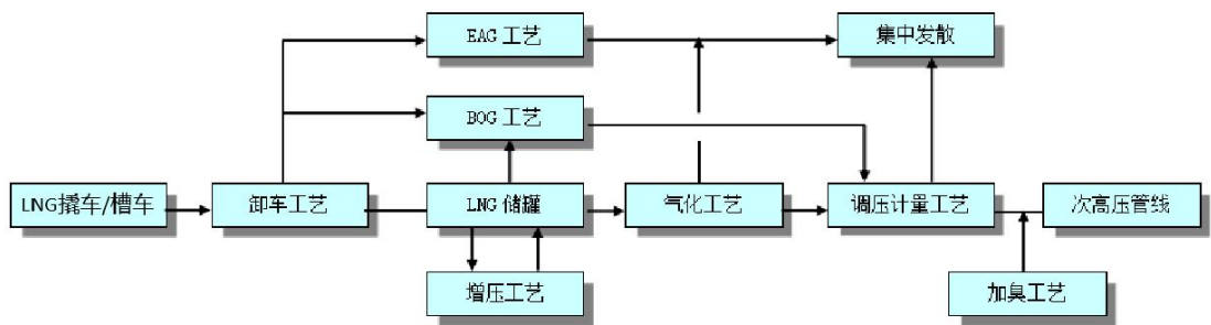
LNG 应急气源站工艺流程
