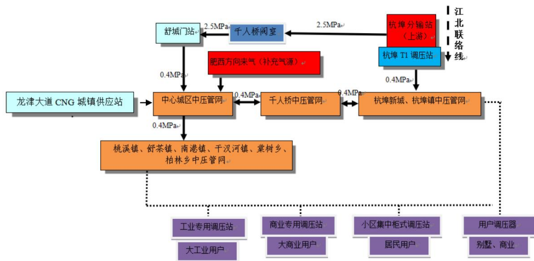
舒城县现状管输气输配系统工艺流程
