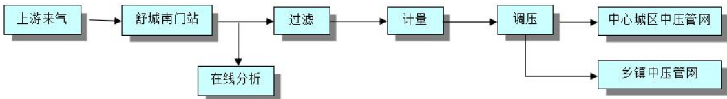
舒城南输气站工艺流程图
