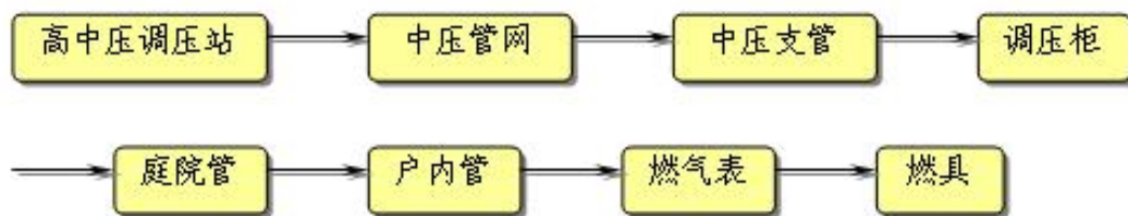
柜式调压流程方框图
