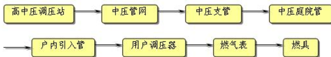
用户调压流程方框图
