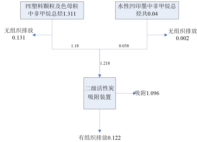
图 2-2 项目非甲烷总烃物料平衡图 单位: t/a
