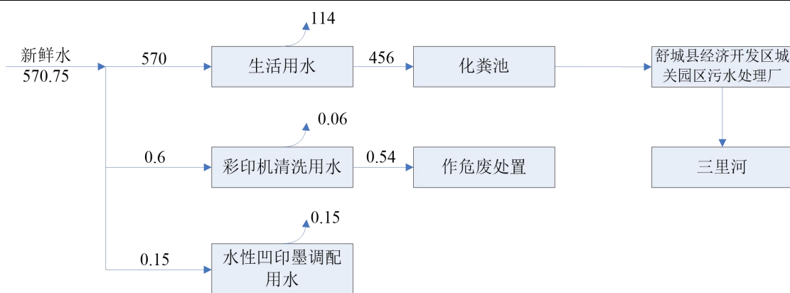
图 2-4 本项目水平衡图 (单位: m³/a)
