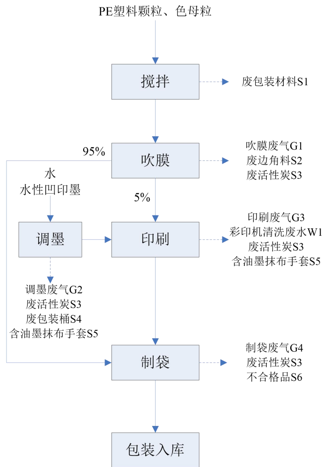
图 2-3 生产工艺流程及产污节点简图
