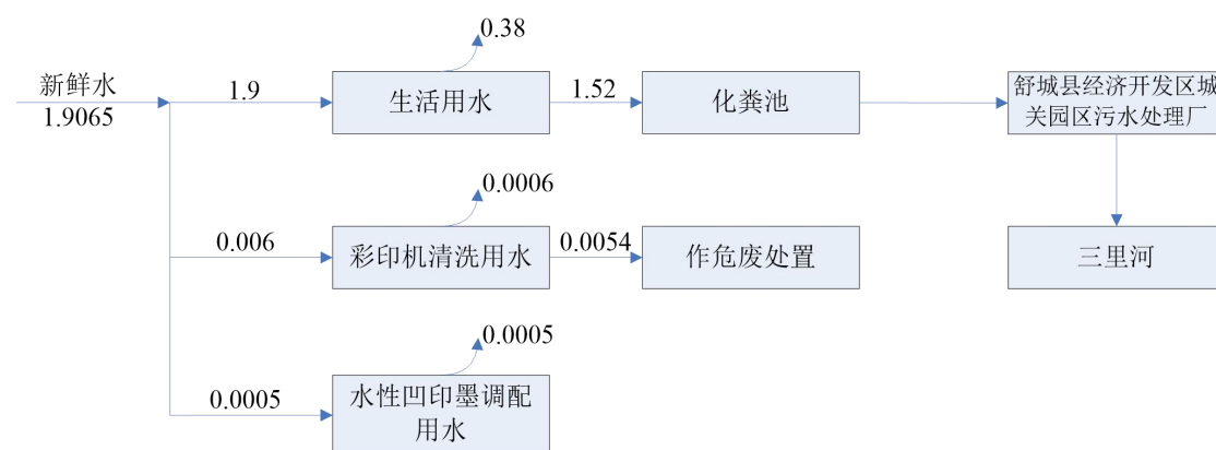
图 2-3 本项目水平衡图 (单位: m 3 /d)
