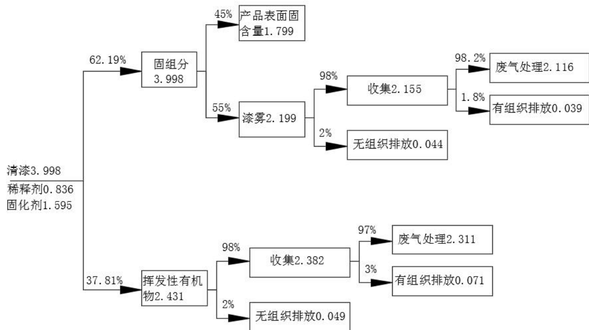
图 2-4 项目运营期清漆物料平衡图 (单位: t/a)
