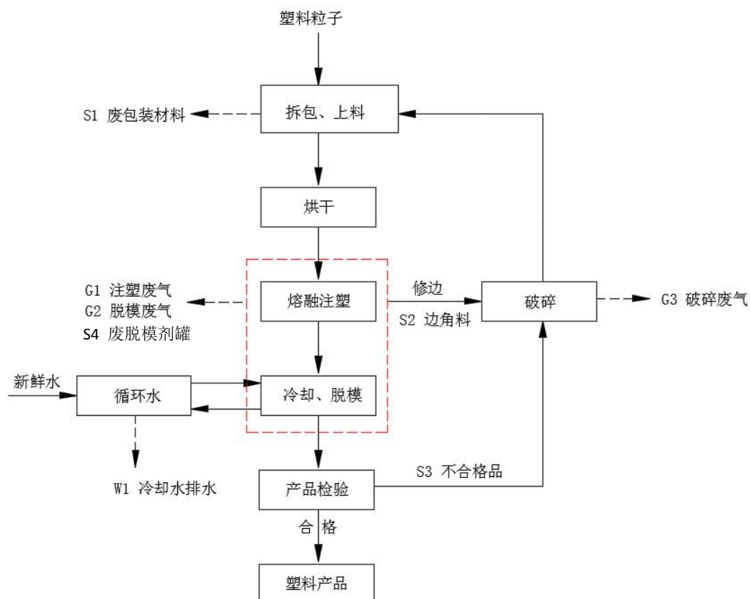
图 2-7 注塑生产工艺流程及产污节点图
