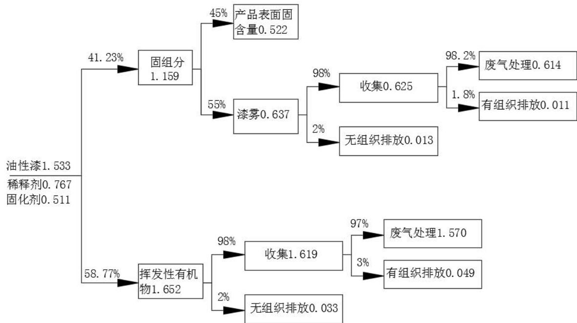
图 2-3 项目运营期油性漆物料平衡图 (单位: t/a)
