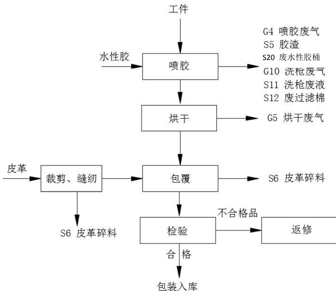
图 2-8 包覆生产工艺流程及产污节点图
