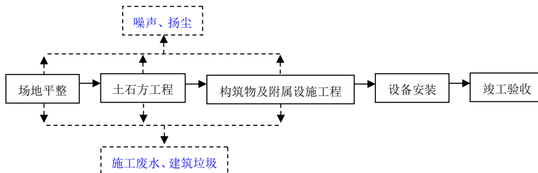
图 2-6 施工期工艺流程及产物环节图
