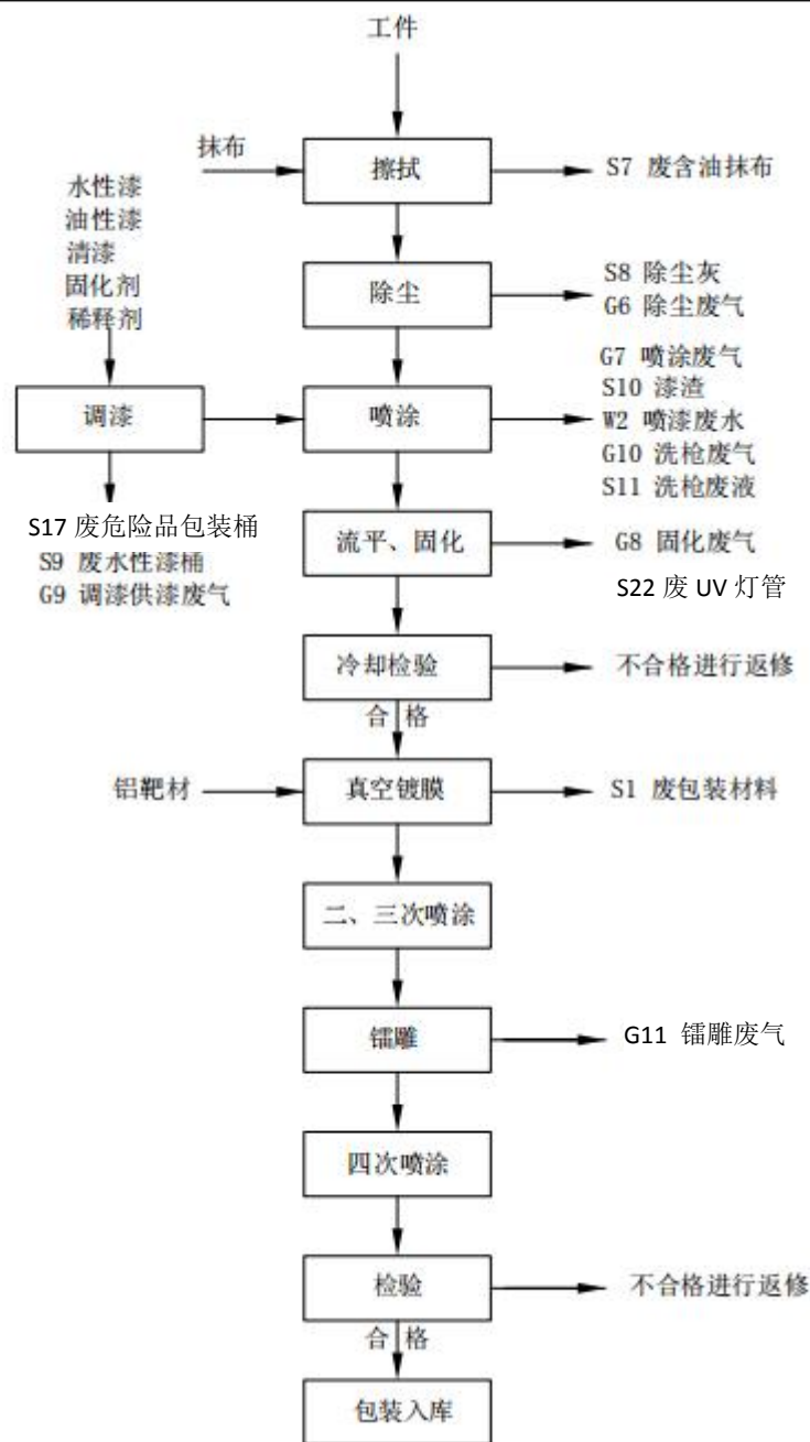
图 2-9 喷涂、镀膜生产工艺流程及产污节点图
