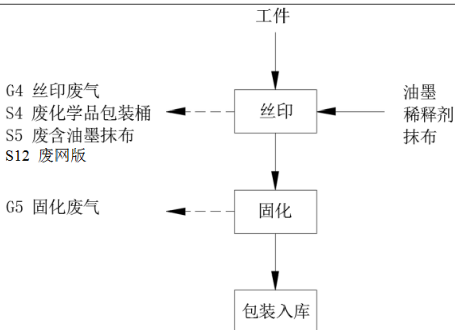
图 2-3 包覆生产工艺流程及产污节点图
