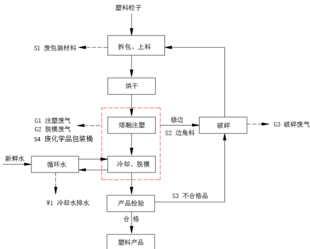
图 2-2 注塑生产工艺流程及产污节点图
