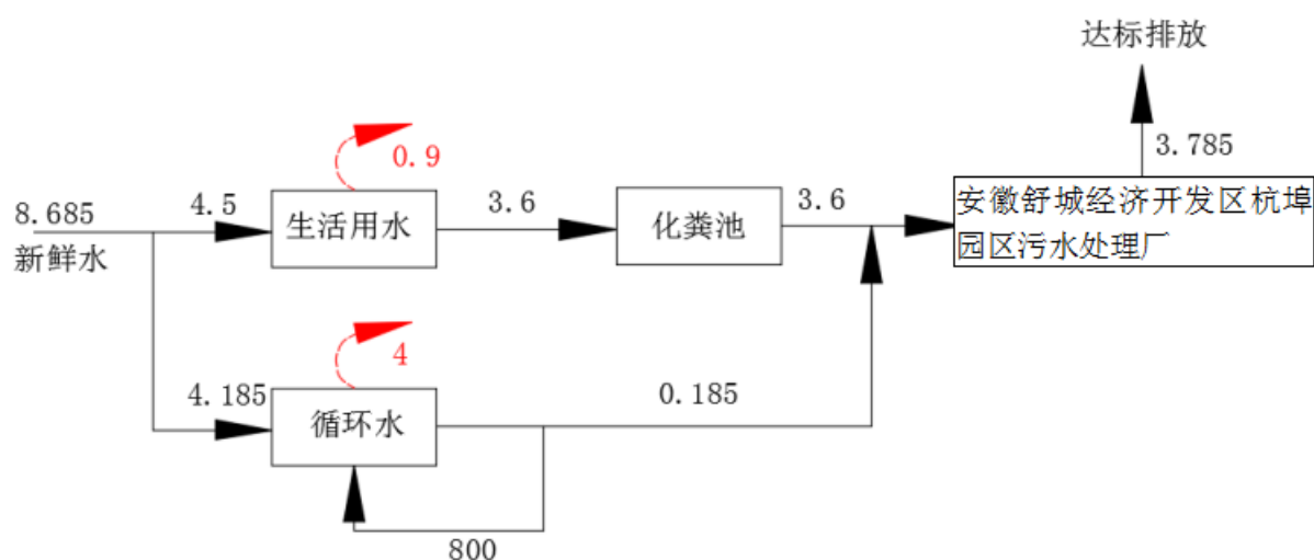
图 2-1 项目水平衡图 (单位: t/d)
